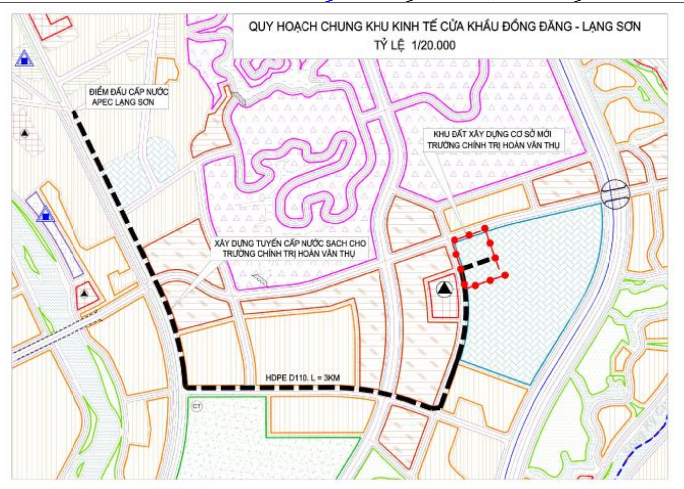
SƠ ĐỒ TUYẾN CẤP NƯỚC CHO DỰ ÁN
