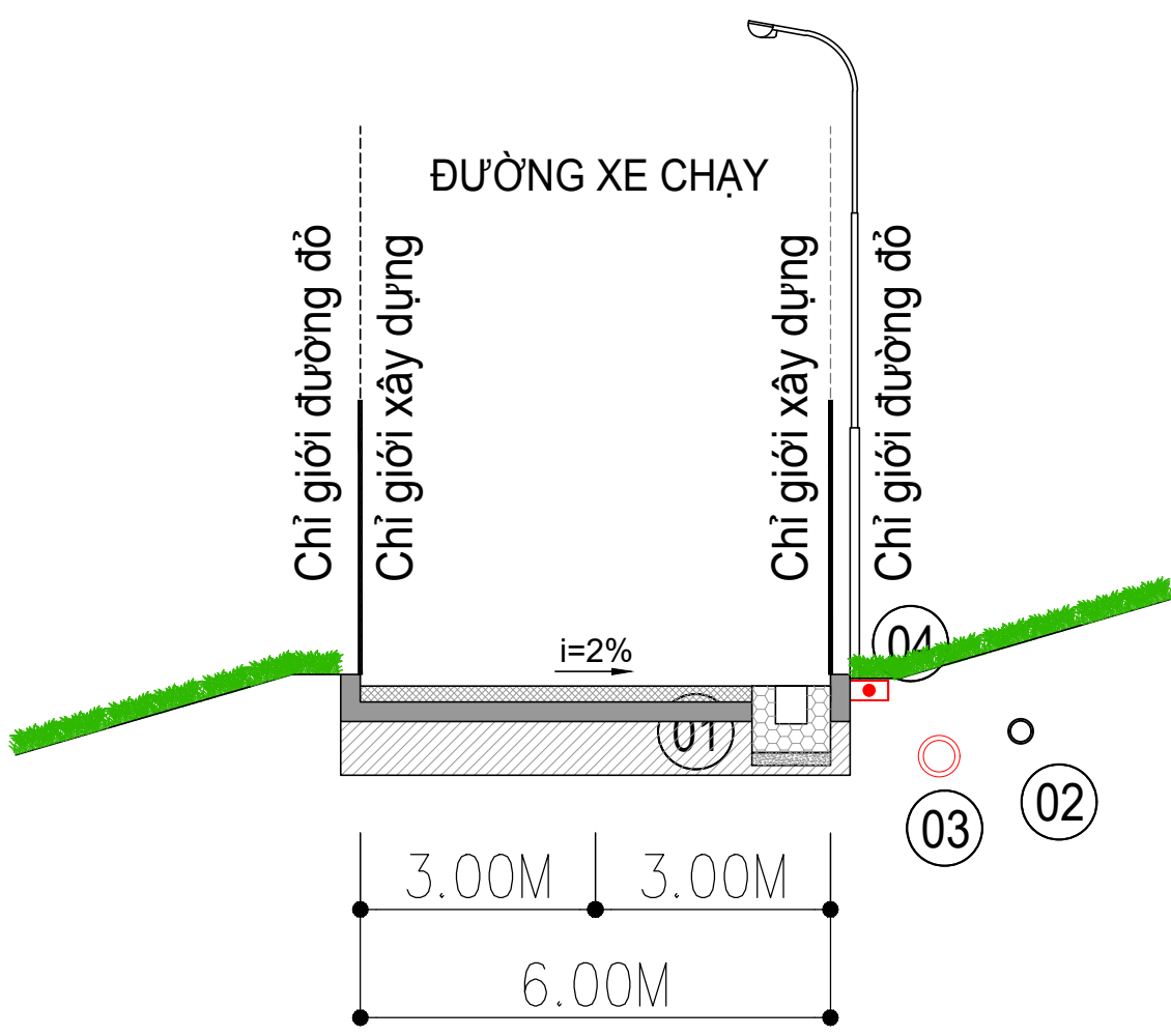
MẶT CẮT 2 - 2
